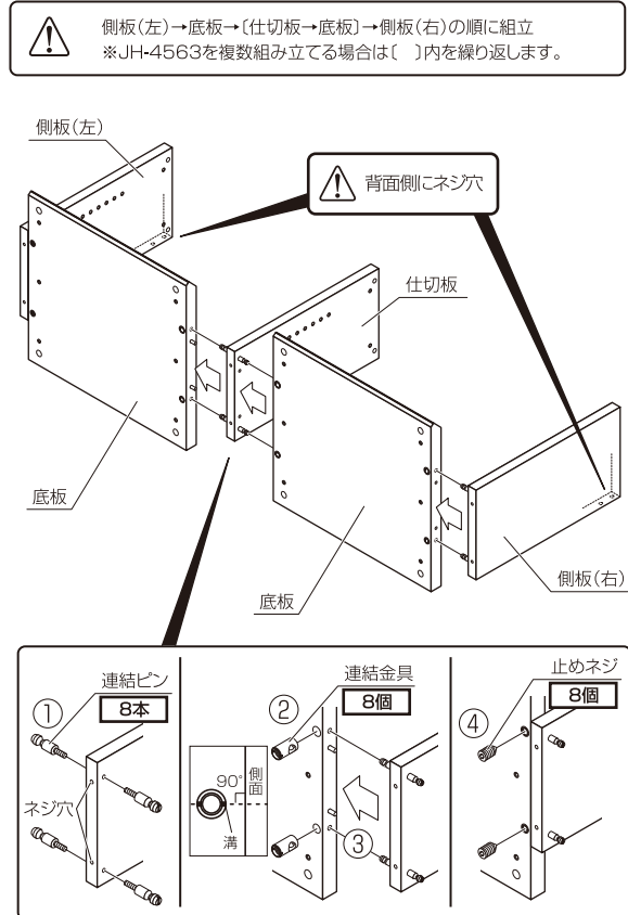
【2連の場合】 J-4560 ×1 JH-4563×1
