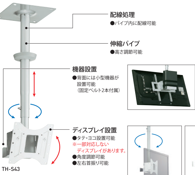
首振り可動イメージ 左右に各70°／前方20°／後方2°
