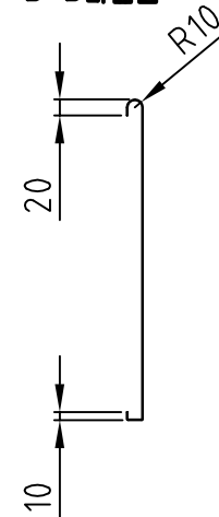
B-B断面図
