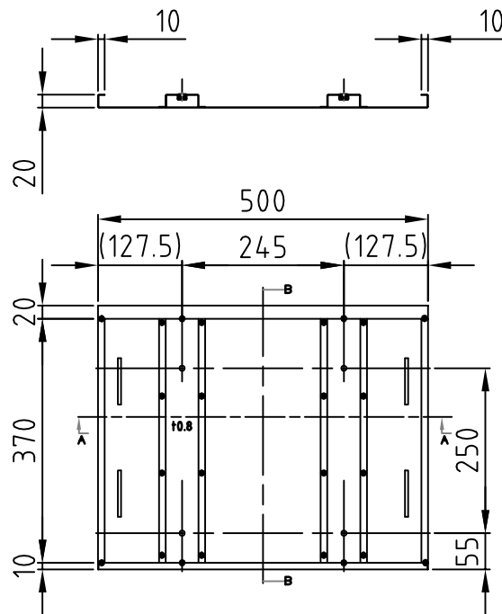
A-A断面図
