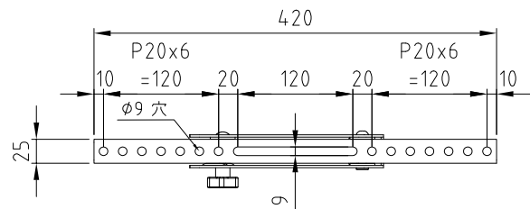
テレビ取付ブラケット 1/5
